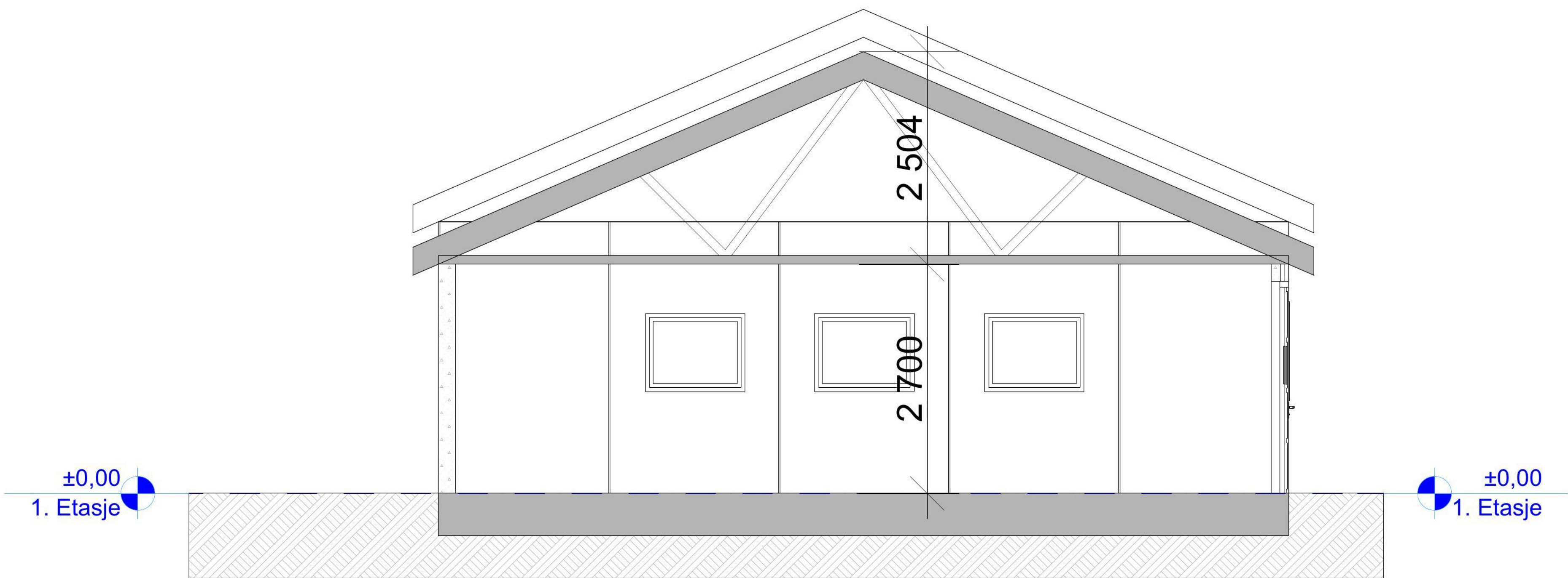
1:50 Snitt A
